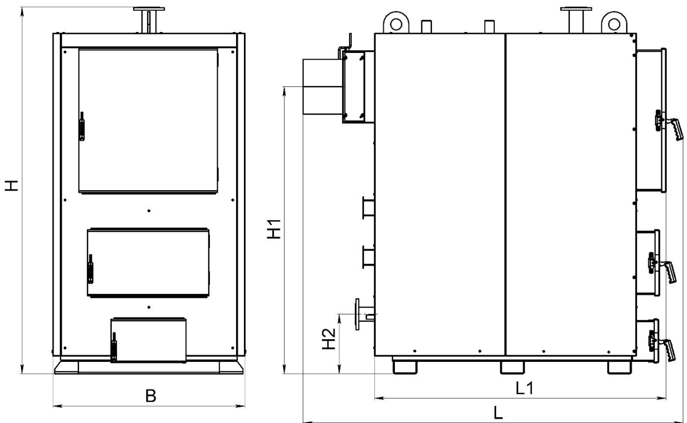
Рисунок 3.1 – Позначення габаритів котла типу КТШ
