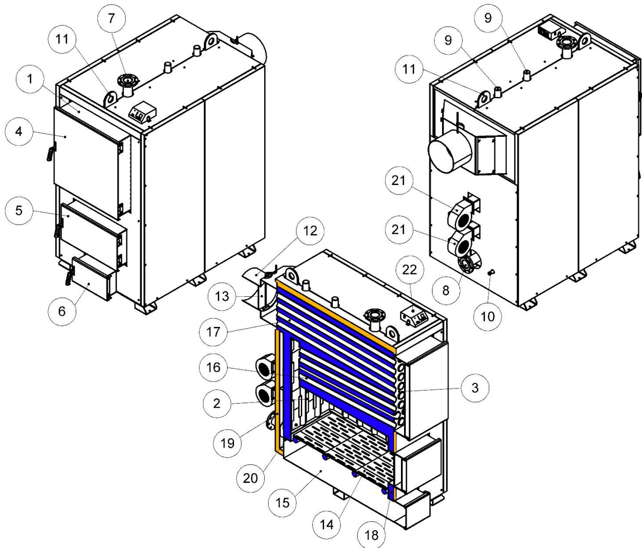
Рисунок 5.1 – Зовнішній вигляд та основні елементи котлів типу КТШ
